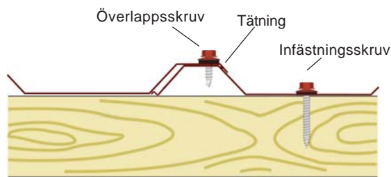
Sidoöverlapp TR35
